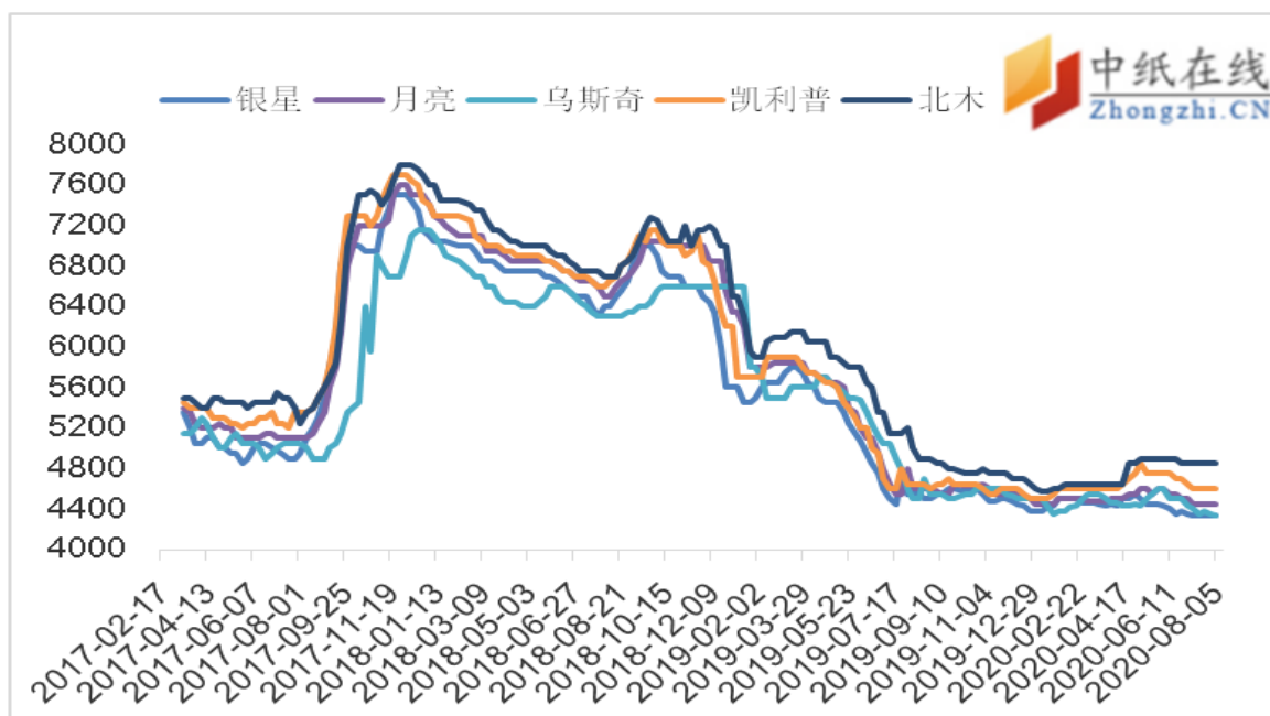
图 3：进口漂针浆现货价格走势
